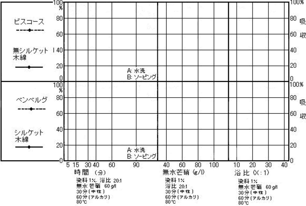
吸 収 曲 線 塩 効 果 曲 線 浴比効果固着曲線
