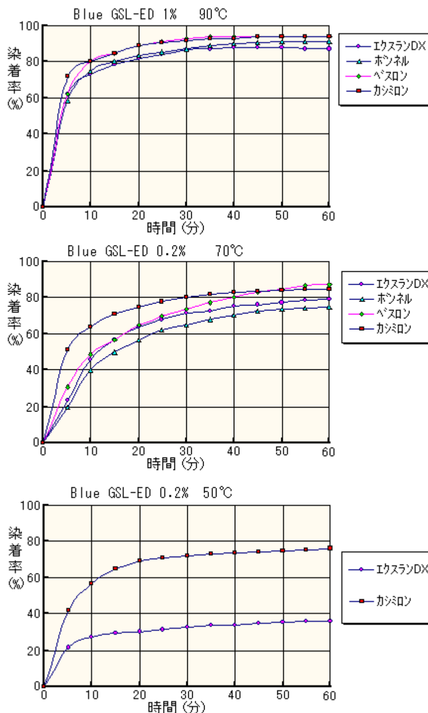
各種繊維における恒温染着曲線
